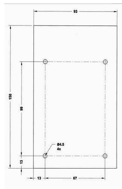
Монтажный шаблон
